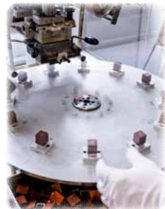
Hubprägemaschine mit automatischem Rundteller.
